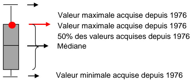
Graphique 2 : Température de fond à Men Er Roué
